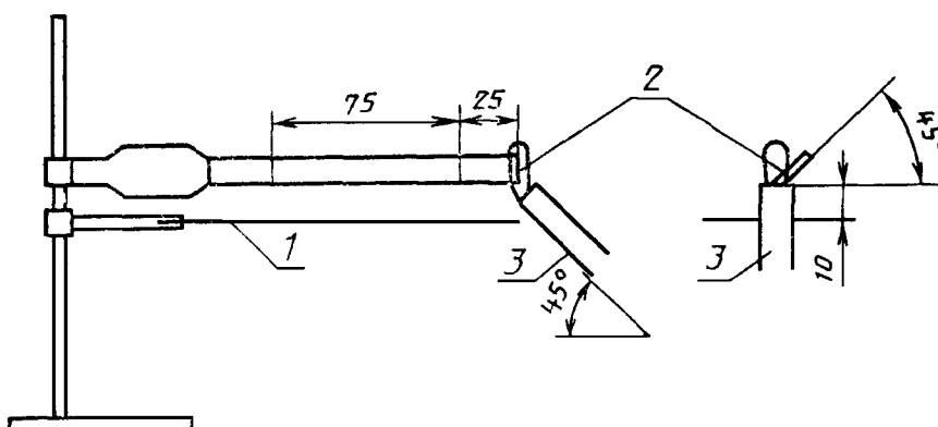
Установка для испытания на горение горизонтально закрепленного образца
